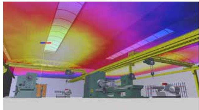
Apport en lumière naturelle des voûtes Ecofil dans un bâtiment industriel
